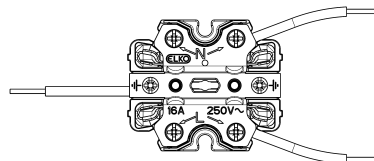
Koblingsskjema
